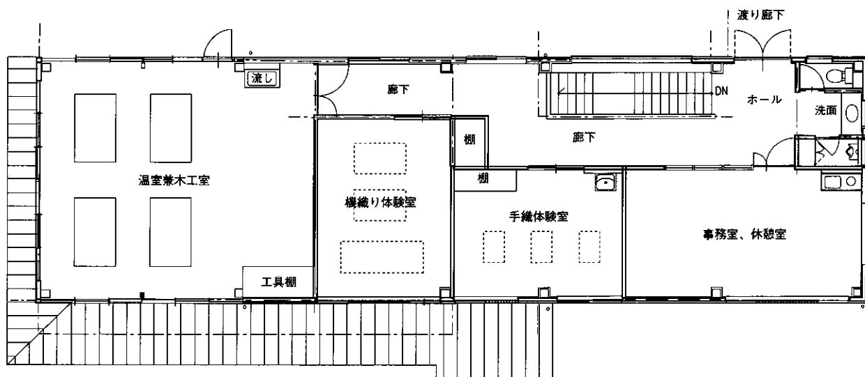
2階平面図
