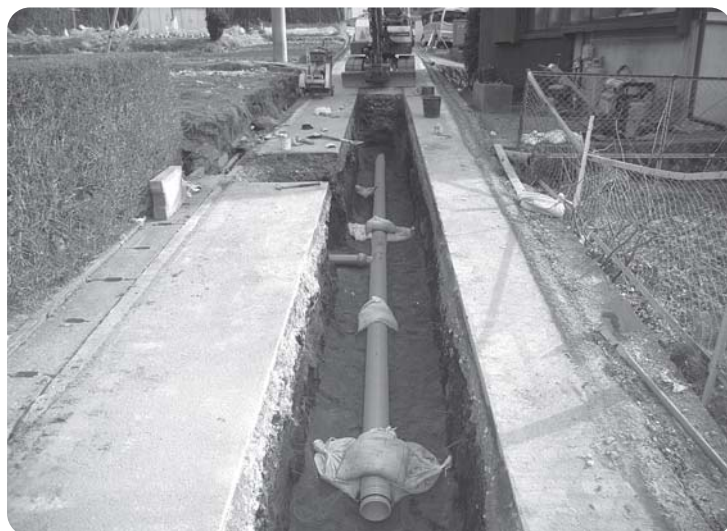
順調に進む倉見区内の下水道工事
