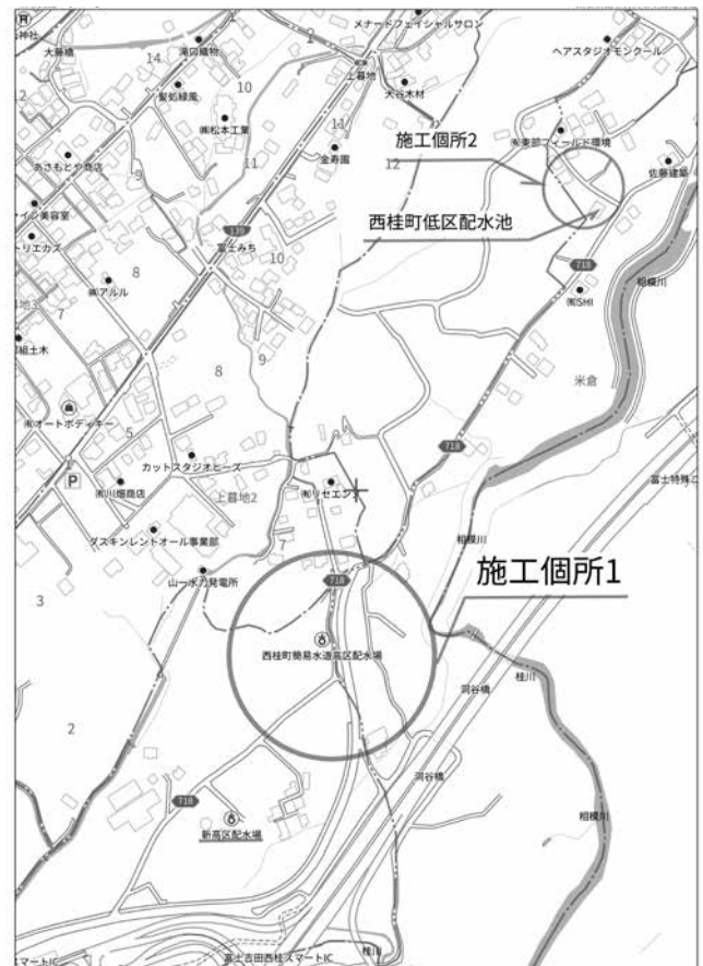
工事図面
